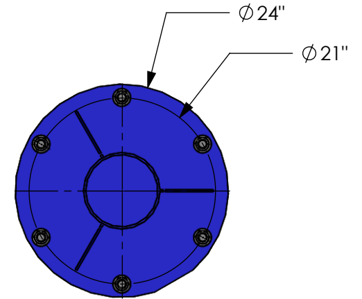
SECTION A-A POSITION DES TROUS DE LA PLAQUE D'ACIER ANCRAGE Ø1" 6X ÉPAISSEUR: 1/2"
