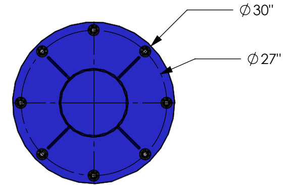
SECTION A-A POSITION DES TROUS DE LA PLAQUE D'ACIER ANCRAGE Ø1" 8X ÉPAISSEUR: 3/4"
