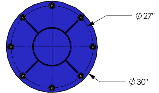
SECTION A-A POSITION DES TROUS DE LA PLAQUE D'ACIER ANCRAGE Ø1" 8X ÉPAISSEUR: 3/4"
