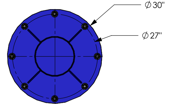
SECTION A-A POSITION DES TROUS DE LA PLAQUE D'ACIER ANCRAGE Ø1" 8X ÉPAISSEUR: 3/4"
