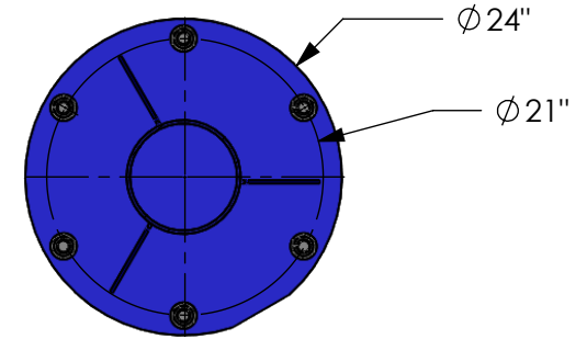
SECTION A-A POSITION DES TROUS DE LA PLAQUE D'ACIER ANCRAGE Ø1" 6X ÉPAISSEUR: 1/2"
