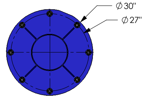
SECTION A-A POSITION DES TROUS DE LA PLAQUE D'ACIER ANCRAGE Ø1" 8X ÉPAISSEUR: 3/4"
