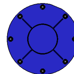
SECTION A-A POSITION DES TROUS DE LA PLAQUE D'ACIER ANCRAGE Ø1" 8X ÉPAISSEUR: 3/4"
