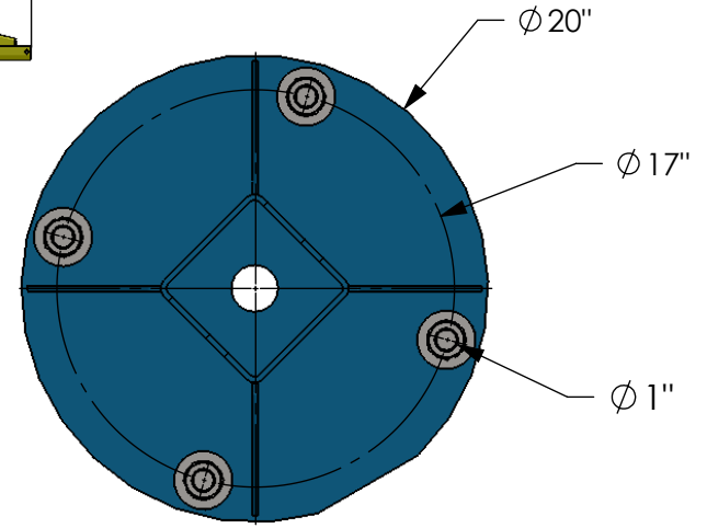
COUPE A-A ÉCHELLE 1 : 9
