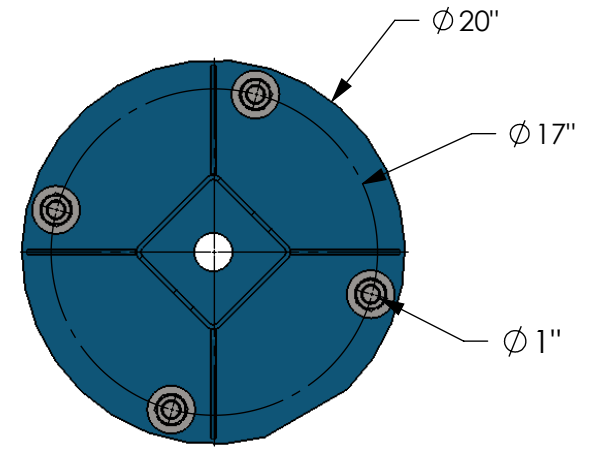
COUPE A-A ÉCHELLE 1 : 10
