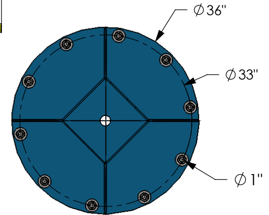
COUPE A-A ÉCHELLE 1 : 18
