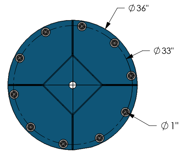
COUPE A-A ÉCHELLE 1 : 16
