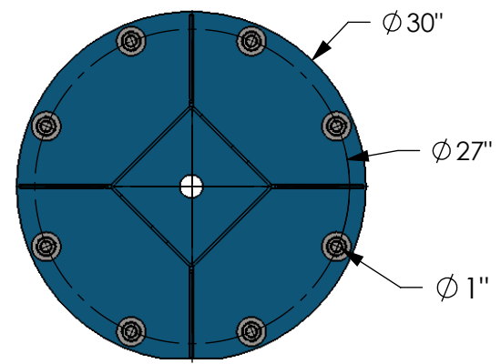
COUPE A-A ÉCHELLE 1 : 15
