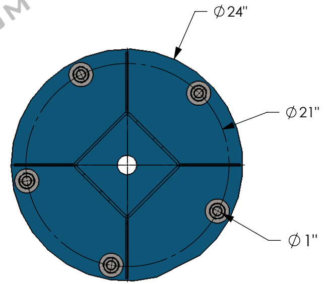
COUPE A-A ÉCHELLE 1 : 10
